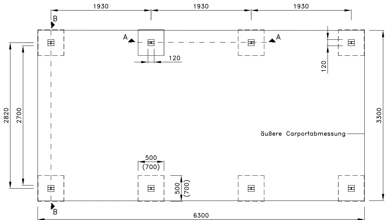
GRUNDRISS
