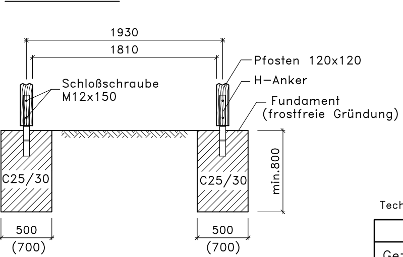
SCHNITT A-A
