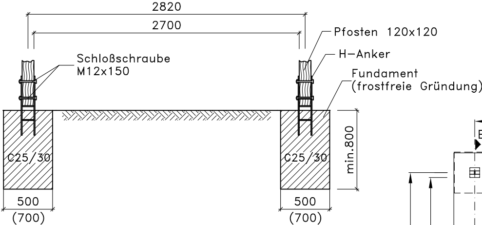
SCHNITT B-B
