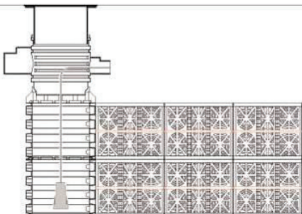
Pumpenschacht
