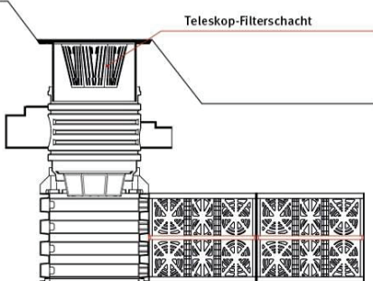
Rigolenüberlaufschacht
