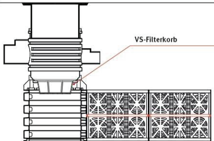
Rigolenüberlaufschacht
