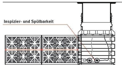
Drosselablaufschacht
