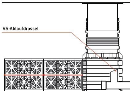
Drosselablaufschacht
