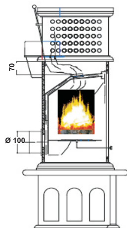
Externer Verbrennungsluftstutzen
