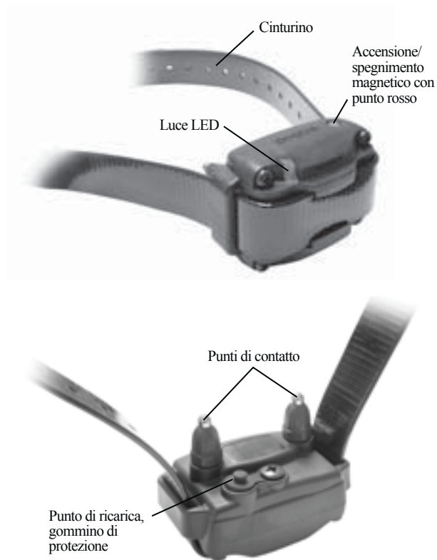
Collare Ricevitore
