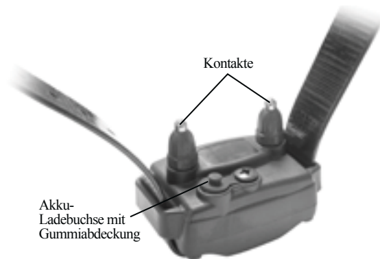
Empfänger
