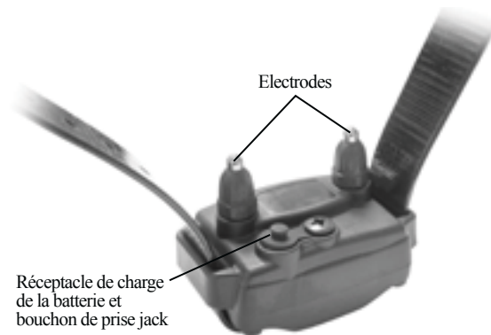
Récepteur
